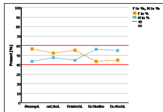
Gleichstellungscontrolling 2008 (Gesamtuniversität)
